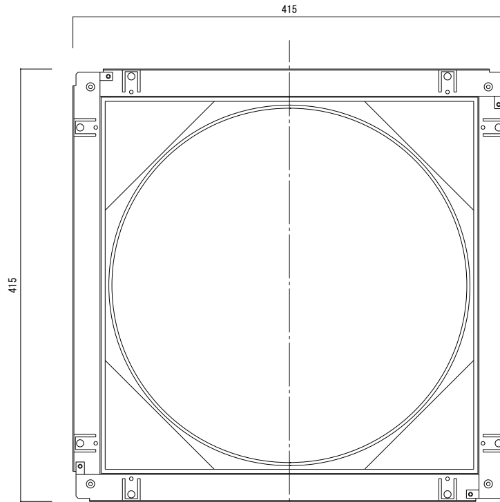
スクエアキット連結ボックス 平面図
