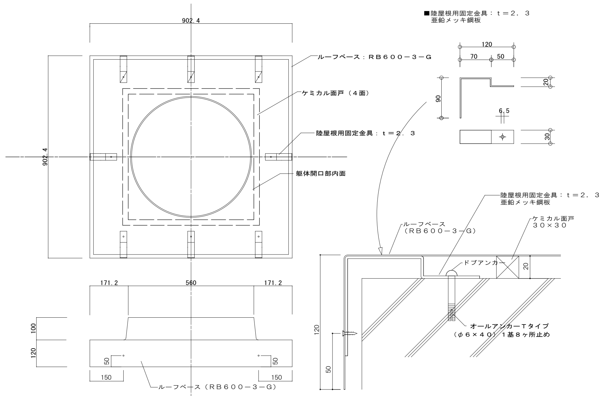
部分詳細図 S = 1 / 2
