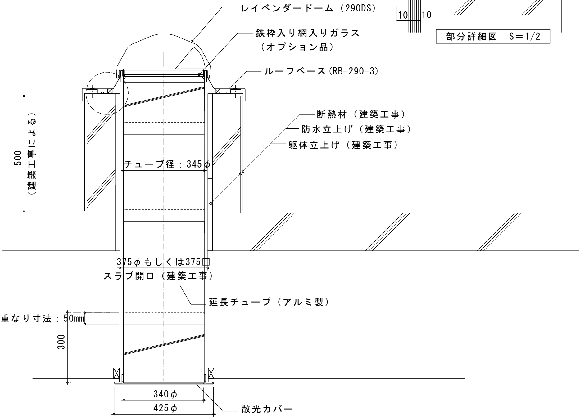
納まり図 (施工例)
