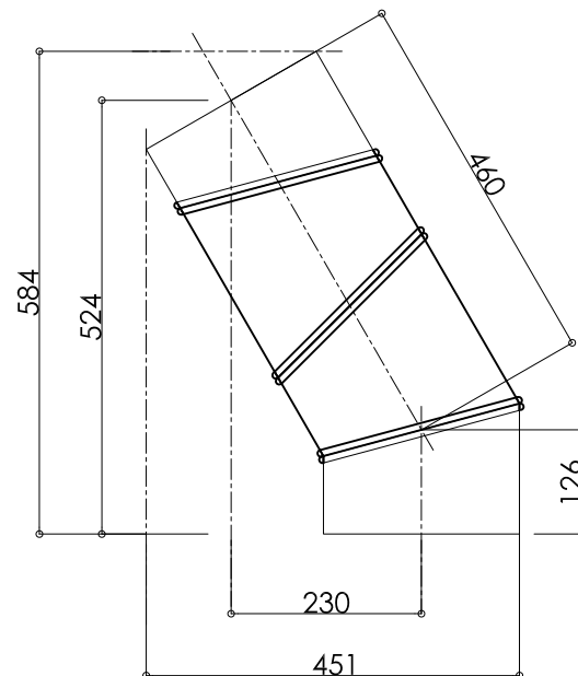
30° アングル SCALE 1:10
