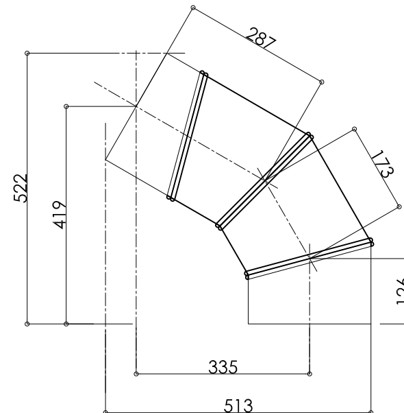
アングル SCALE 1:10
