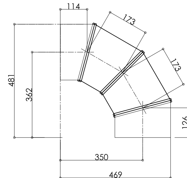
90° アングル SCALE 1:10
