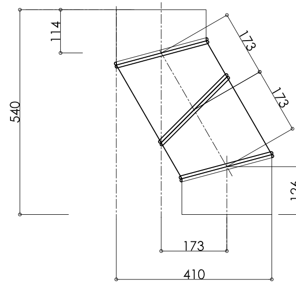
アングル SCALE 1:10
