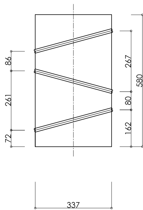
ストレート SCALE 1:10
