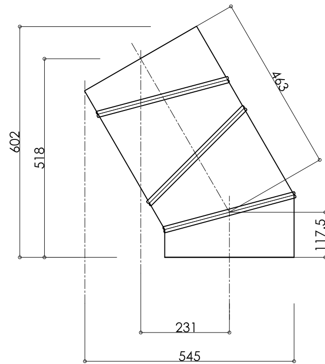
30°アングル SCALE 1:10
