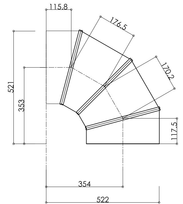
90°アングル SCALE 1:10
