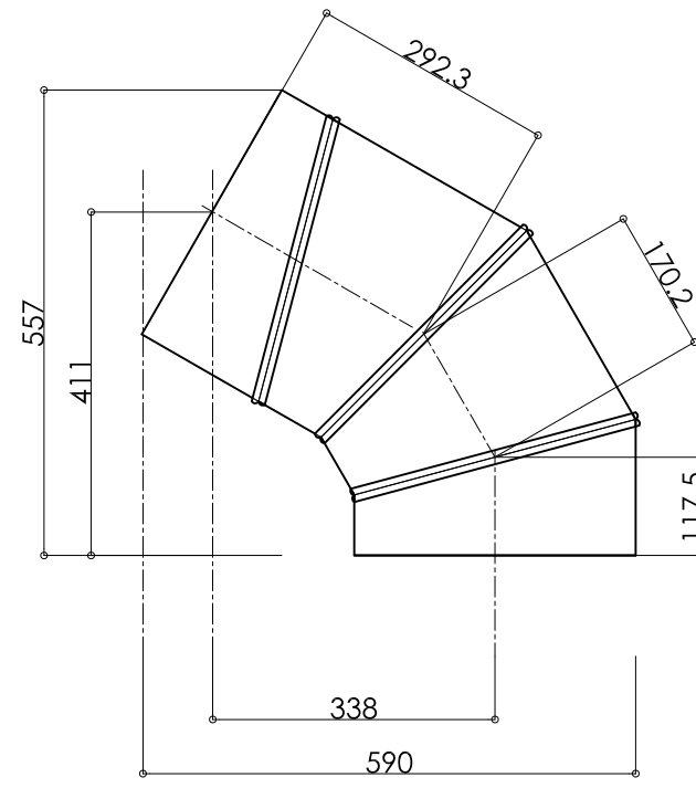
60°アングル SCALE 1:10
