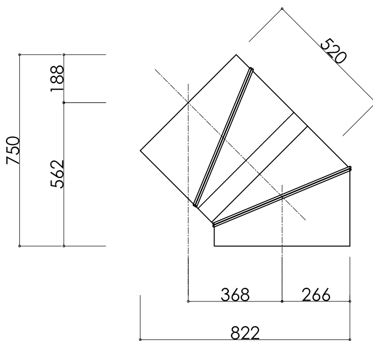
45° アングル SCALE 1:15
