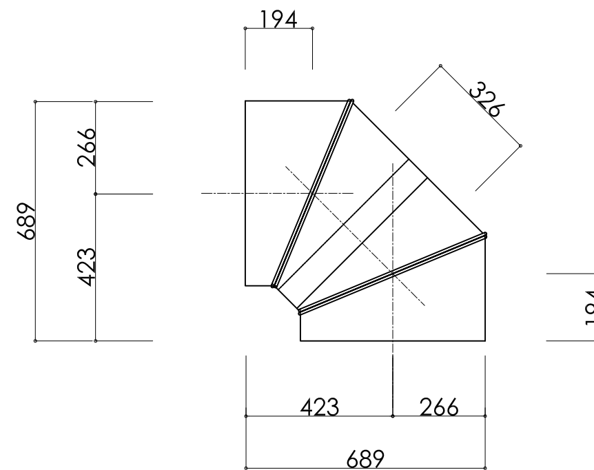
90° アングル SCALE 1:15
